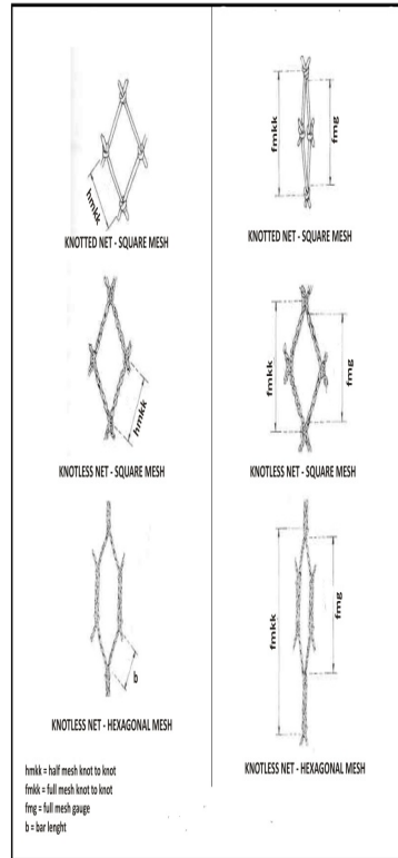
الشكل 3: أشكال عيون الشبكة وأنواع العقد
