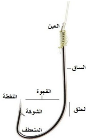
الشكل 23: شكل الخطاف و مكوناته
